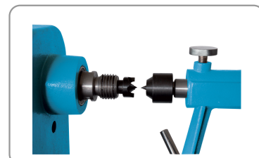
Broche entraînement cm2 fileté m33 x 3,5 mm
