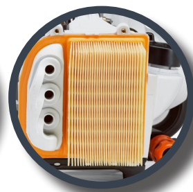
Système de filtration nécessitant peu d'entretien grâce à la pré-séparation cyclonique
